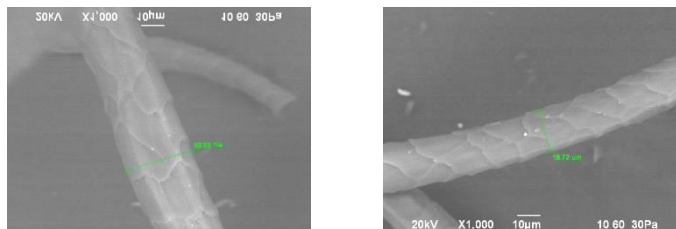
Рис. 5. Микроструктура мериносовых волокон (увеличение \times 1000 )
