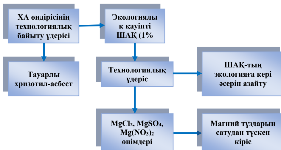
Сурет 1. Магний тұздарын алу және оның қоршаған ортаға зиянды әсерін азайтуға бағытталған ШАҚ-ты қайтаөндеудің технологиясының принципіалды схемасы
